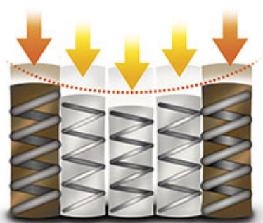
Molle a sostegno differenziato inserite all'interno di sacchetti microforati
