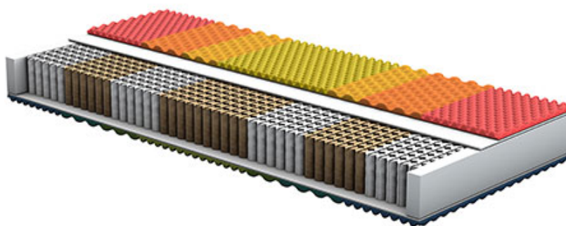
Materasso con 800 molle a 4 strati sovrapposti e 2 soluzioni di riposo lato Memory e lato Waterflex
